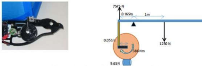
Fig:6.1.Kestrel Ornithopter
